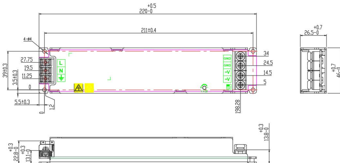
外形尺寸及安装孔——端子坐标图
