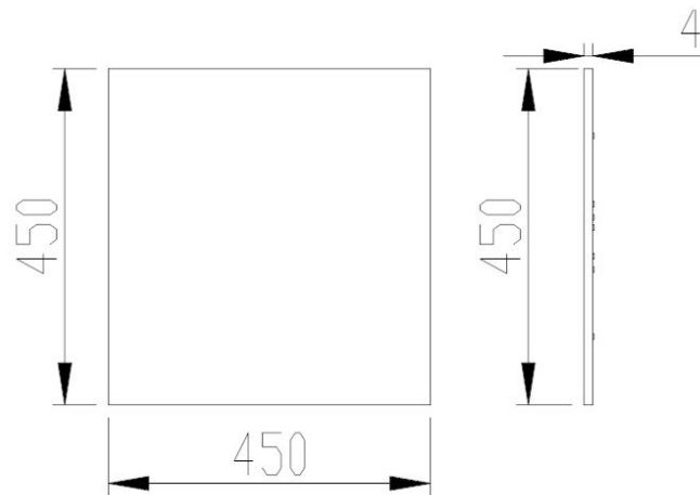
图4 铝散热板尺寸图
